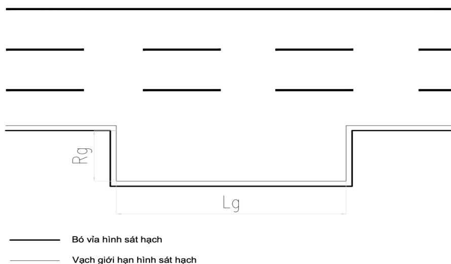
Hình 14: Hình bài sát hạch ghép xe ngang vào nơi đỗ đối với hạng C, D1, D2, D
