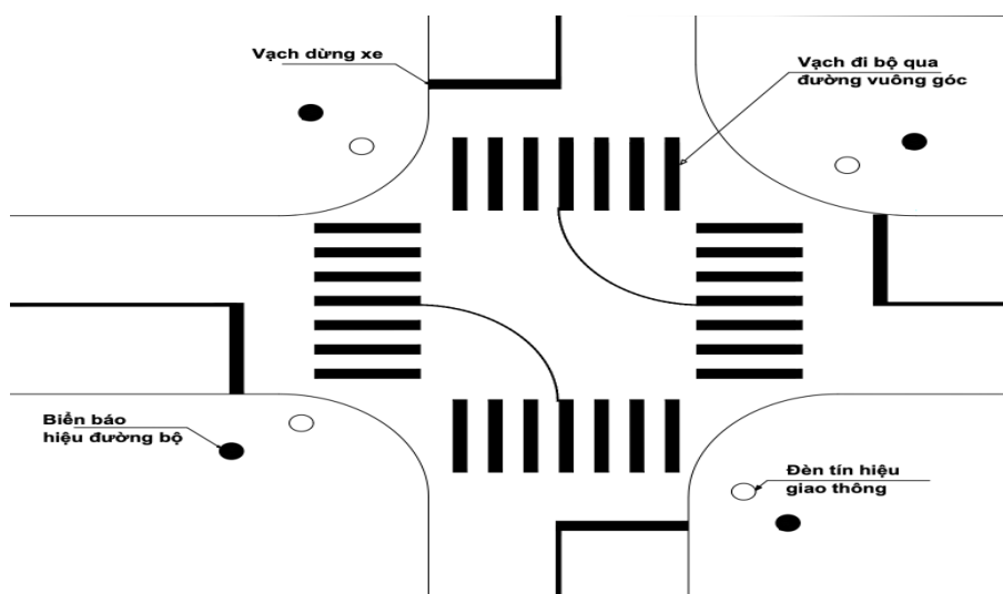
Hình 10: Hình bài sát hạch qua ngã tư
