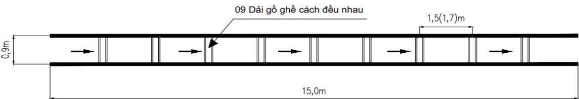
TIẾT DIỆN DẢI GỒ GHỀ HẠNG A1 - A
