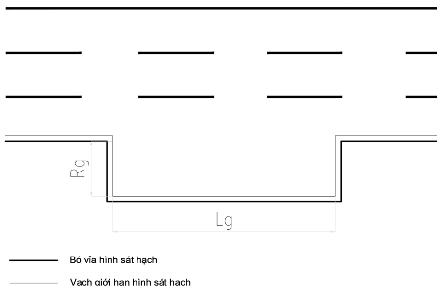
Hình 13: Hình bài sát hạch ghép xe ngang vào nơi đỗ đối với hạng B
