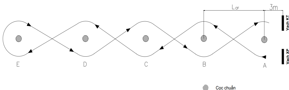
Hình 17: Hình bài sát hạch đi qua 05 cọc chuẩn hạng BE, D1E, D2E, DE
