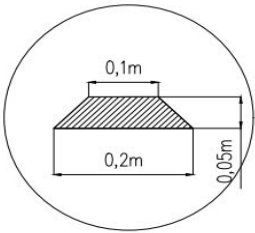
TIẾT DIỆN DẢI GỒ GHỀ HẠNG A1 - A
