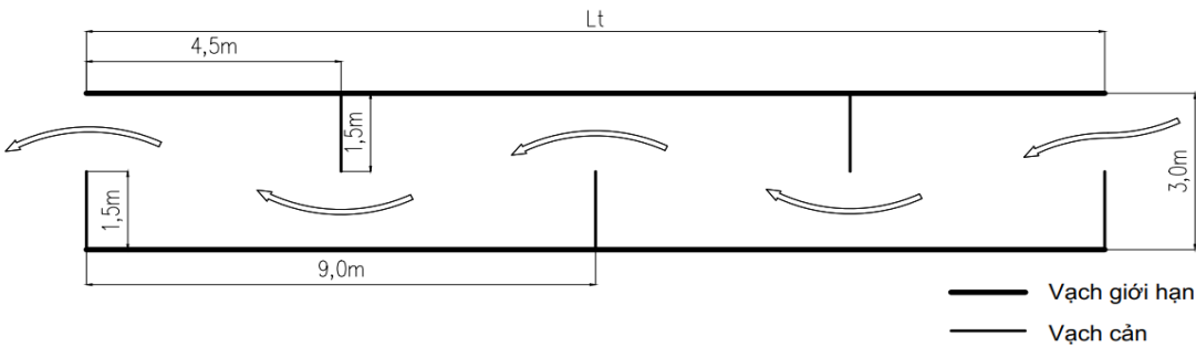
Hình 3: Hình bài sát hạch đường có vạch căn
