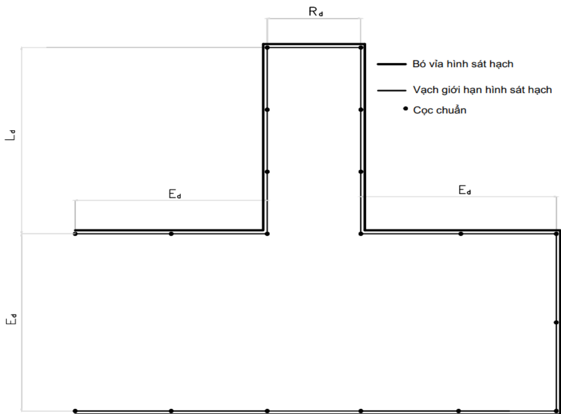
Hình 19: Hình bài sát hạch ghép xe dọc vào nơi đỗ hạng C1E, CE
