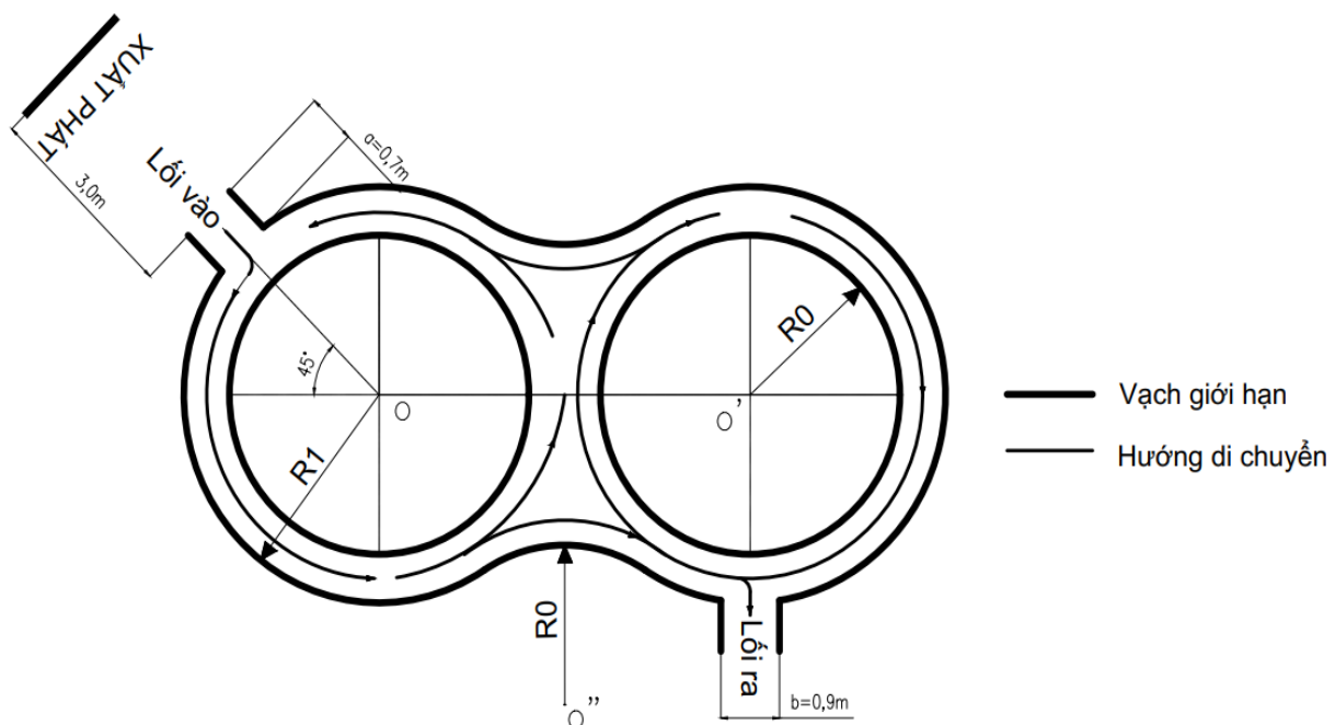
Hình 1: Hình bài sát hạch hình số 8
