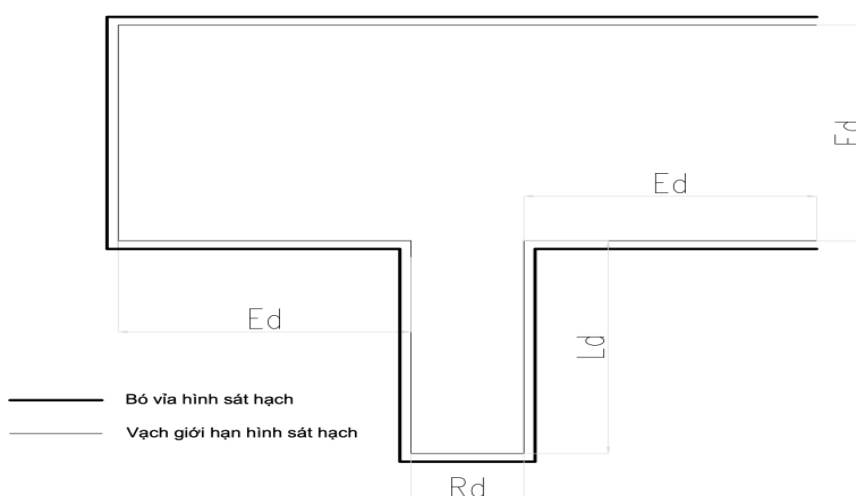
Hình 12: Hình bài sát hạch ghép xe dọc vào nơi đỗ đối với hạng B và hạng C1
