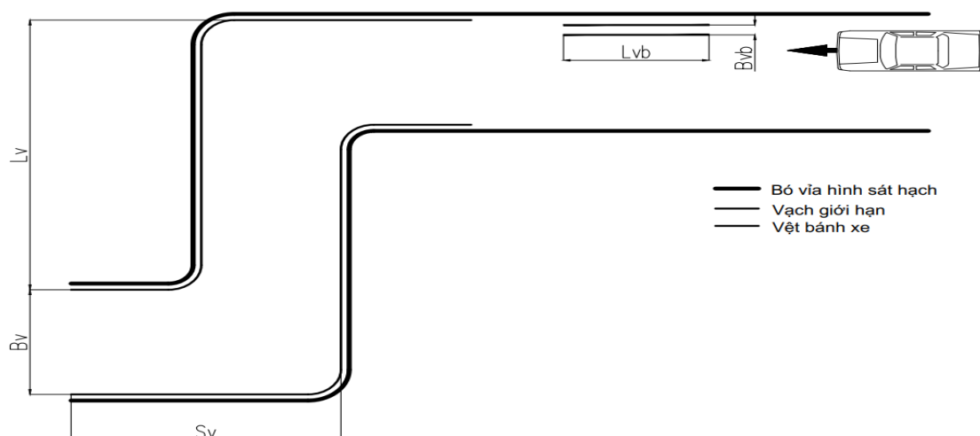
Hình 9: Hình bài sát hạch qua vệt bánh xe và đường vòng vuông góc
