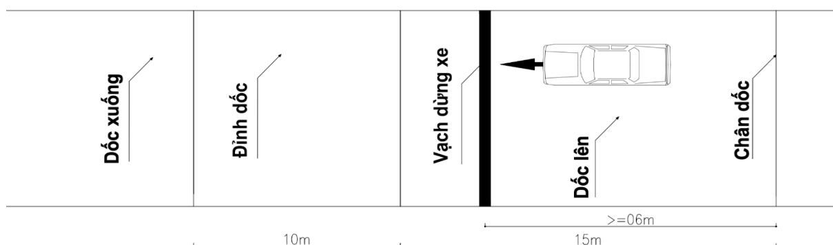
Hình 8: Hình bài sát hạch dừng và khởi hành xe trên dốc
